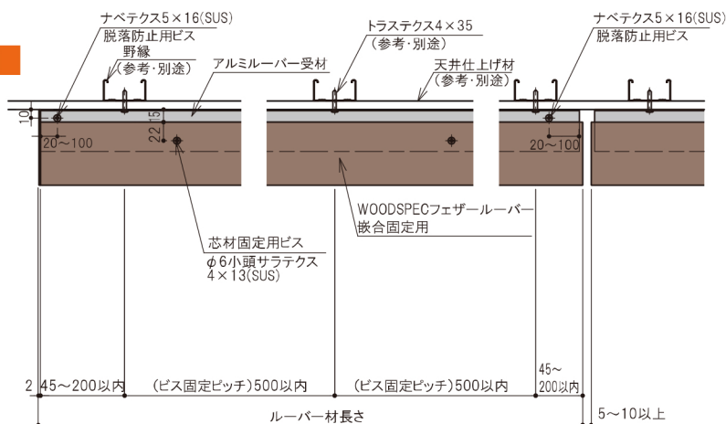
水平断面図
