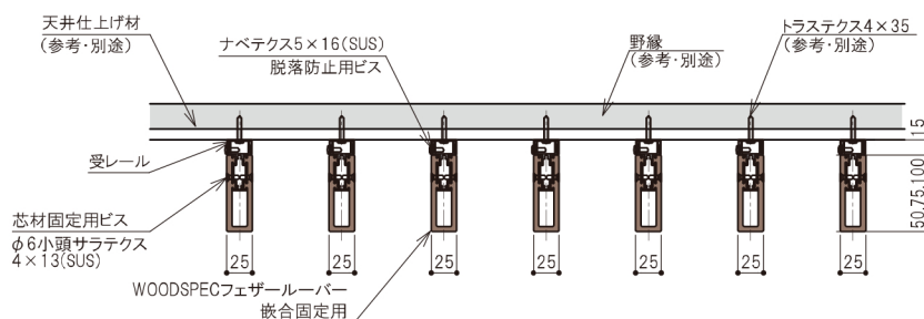
正面図
